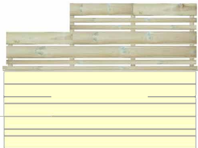
Kombination vindskydd/insynsskydd
